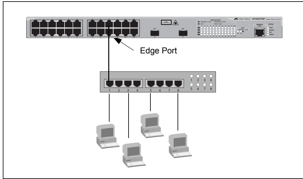
Figure 23. Edge Port
